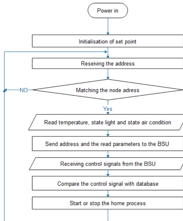
Fig. 25 first SU flowchart.
