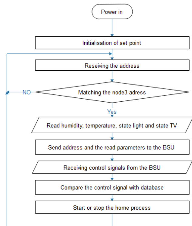
Fig. 27 third SU flowchart.
