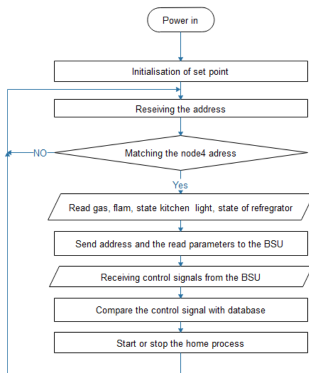
Fig. 28 forth SU flowchart.
