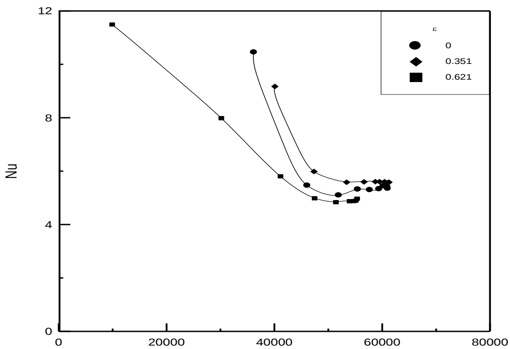
شكل (8) توزيع معدل عدد نسلت مع عدد رالي للموقع الزاوي ( \delta=180^\circ )
