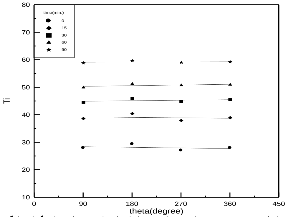
شكل (5) توزيع درجات الحرارة على محيط السطح الخارجي للأسطوانة الداخلية
