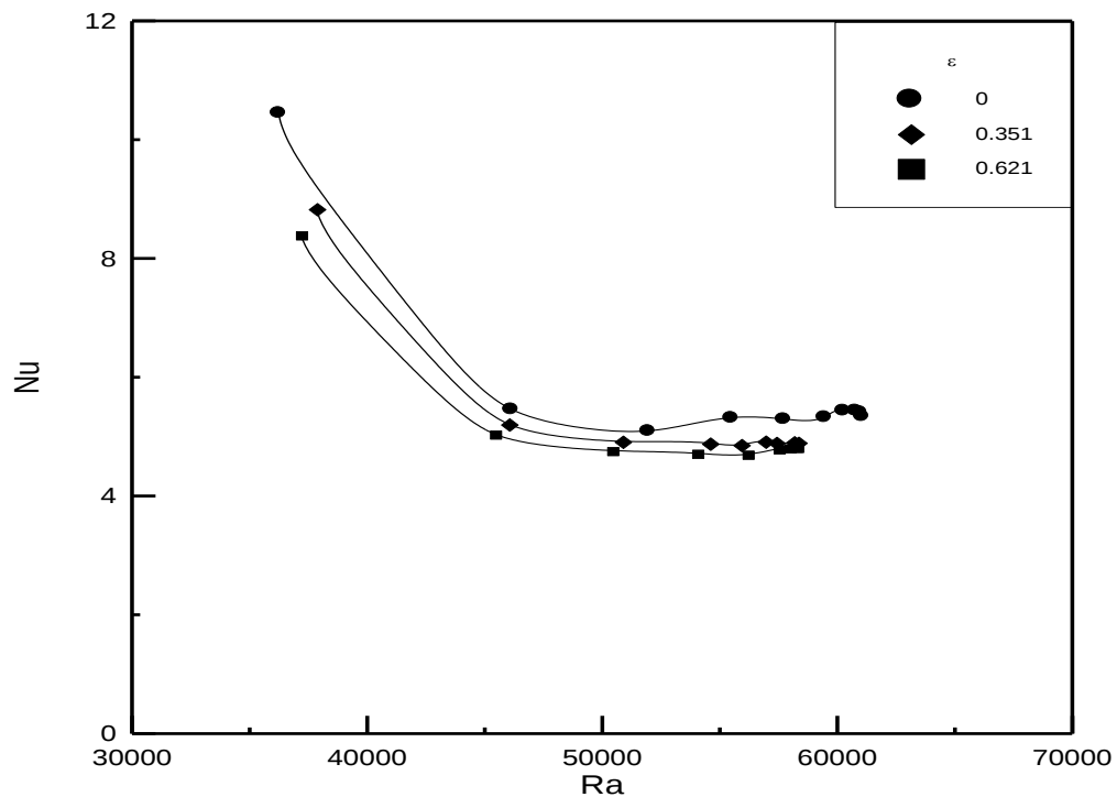
شكل (7) توزيع معدل عدد نسلت مع عدد رالي للموقع الزاوي ( \delta=90^\circ )
