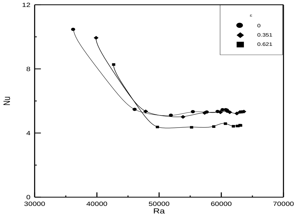
شكل (6) توزيع معدل عدد نسلت مع عدد رالي للموقع الزاوي ( \delta=0^\circ )
