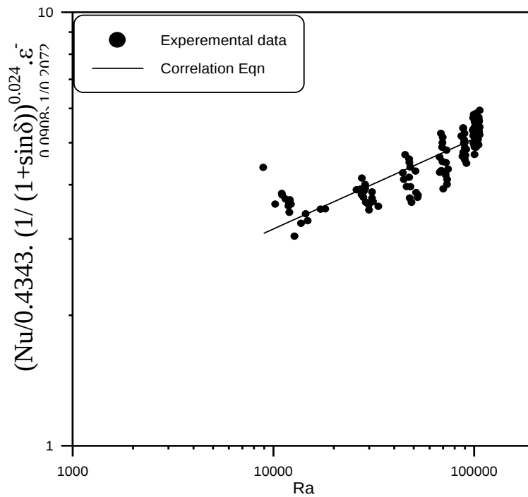
شكل (9) نتائج انتقال الحرارة مع المعادلة الارتباطية
