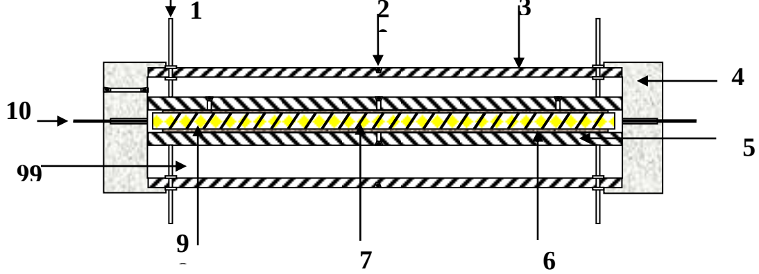
شكل (2) الرسم التخطيطي للمنشأ التجريبي المستخدم في الاختبار
