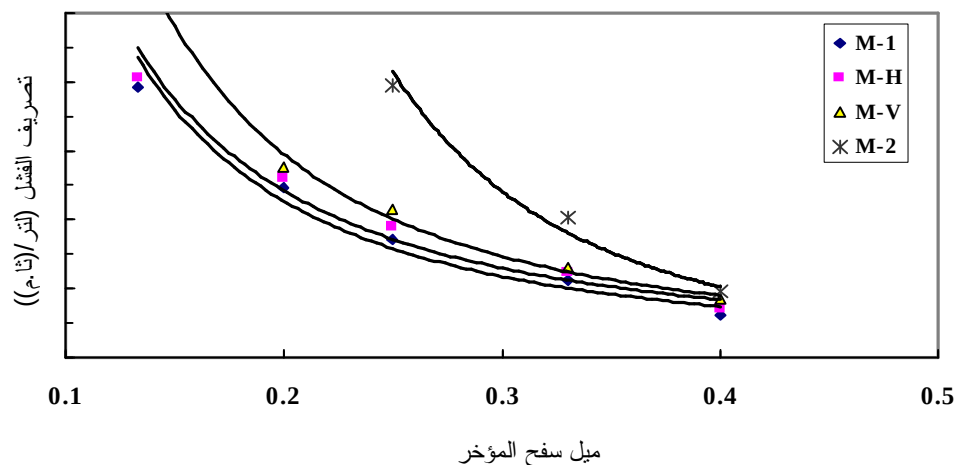
الشكل (5ب): العلاقة بين تصريف الفشل وميل سفح المؤخر لكتلة السلة الصخرية (1.220) كغم
