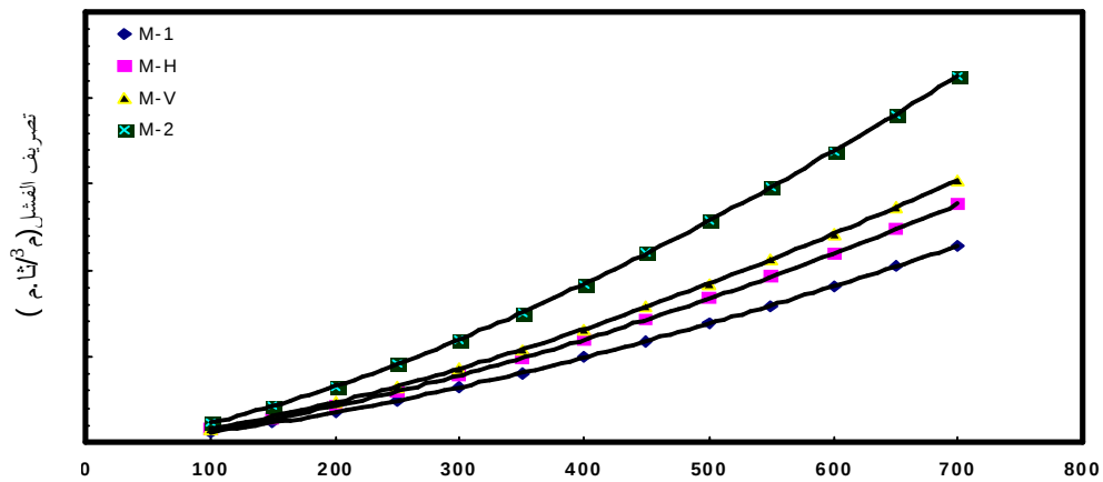
الشكل (6 د): العلاقة بين تصريف الفشل وكتلة السلة الصخرية للميل (1V:5H)
