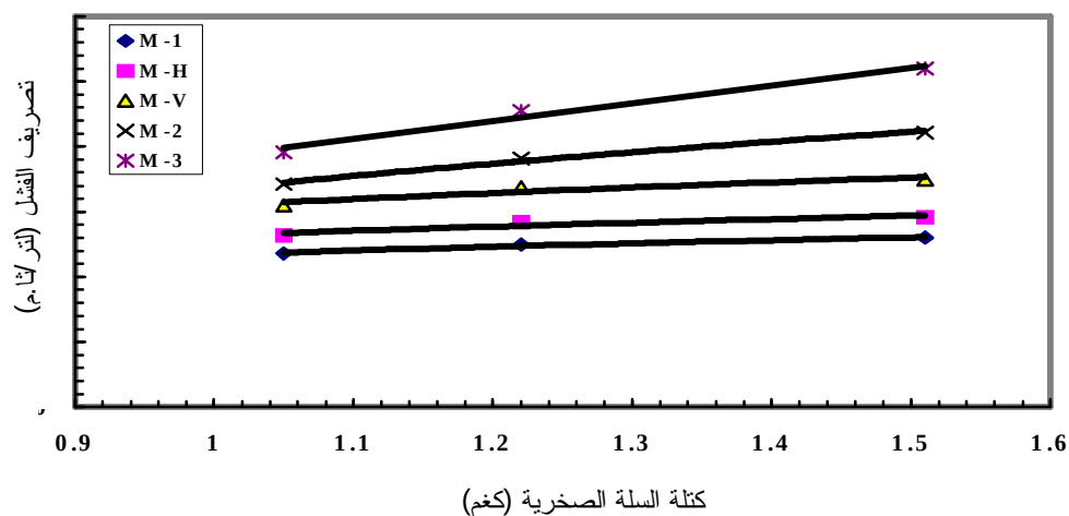
الشكل (5ج): العلاقة بين تصريف الفشل وميل سفح المؤخر لكتلة السلة الصخرية (1.05) كغم
