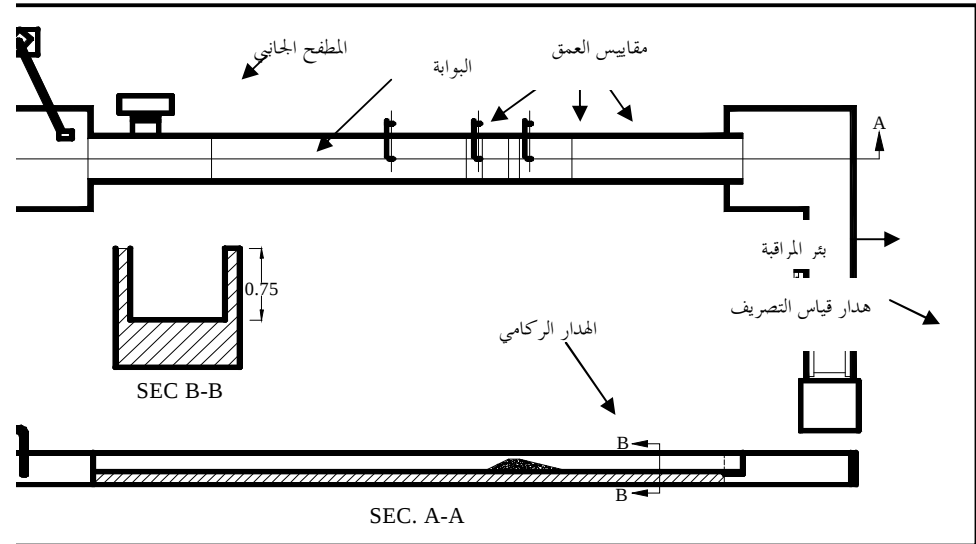
الشكل (2) : مقطع طولي للهدار الركامي
