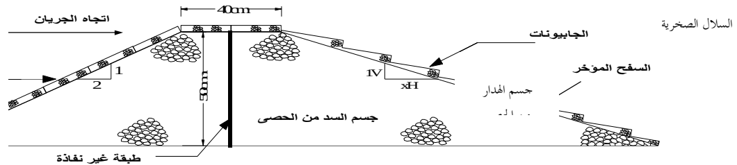
مقطع طولي للسد الركامي الغاطس
