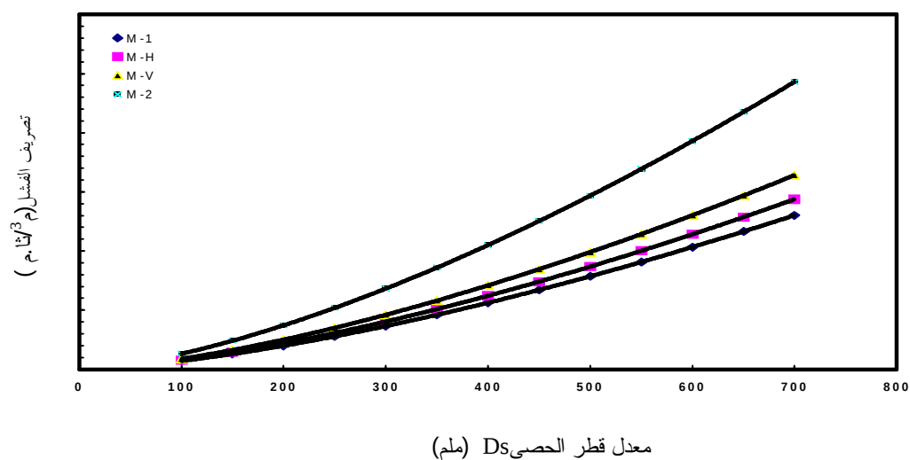
الشكل (7د): المنحنى التصميمي للعلاقة بين تصريف الفشل ومعدل قطر الحصى لحالات الوضع الأربعة للميل (1V:5H).
