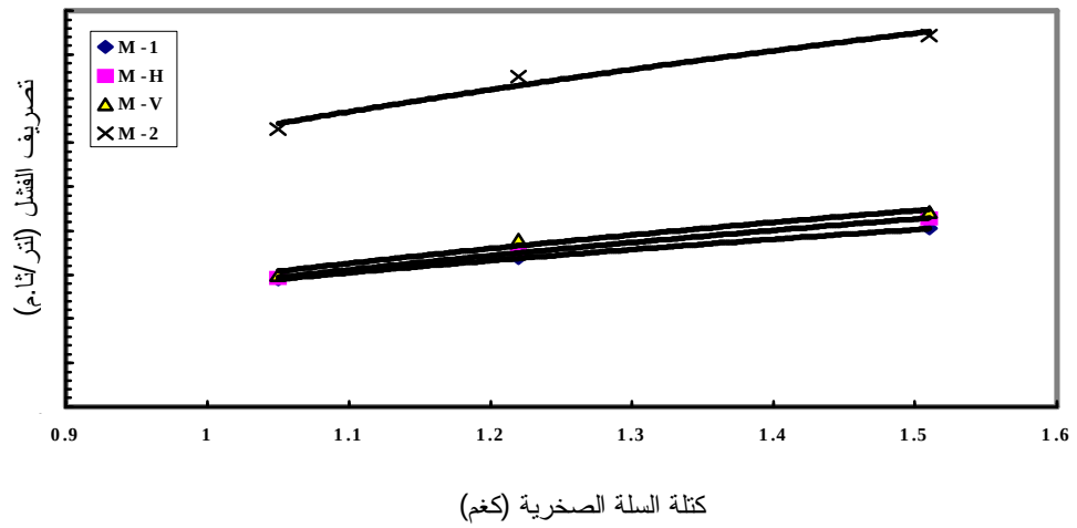
الشكل (6 ج): العلاقة بين تصريف الفشل وكتلة السلة الصخرية للميل (1V:4H)
