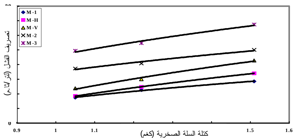
الشكل (6 أ): العلاقة بين تصريف الفشل وكتلة السلة الصخرية للميل (1V:2.5H)
