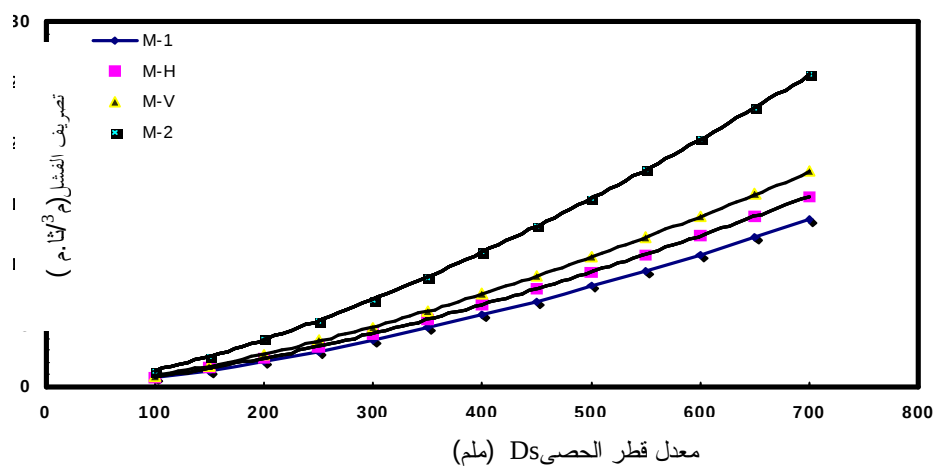
الشكل (7جـ): المنحنى التصميمي للعلاقة بين تصريف الفشل ومعدل قطر الحصى لحالات الوضع الأربعة للميل (1V:4H).
