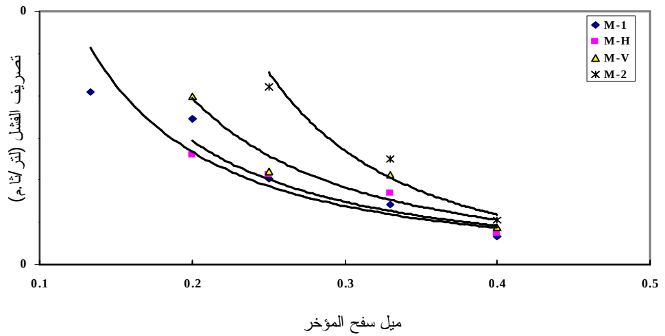
الشكل (4): شكل سطح الماء للميل (1V:4H) والربط (M-H) وكتلة السلة الصخرية (1.22) كغم
