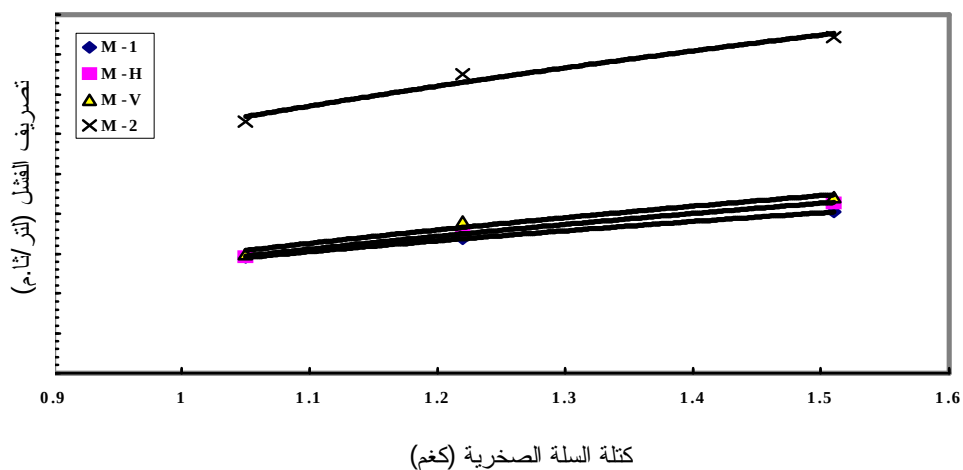
الشكل (6 ب): العلاقة بين تصريف الفشل وكتلة السلة الصخرية للميل (1V:3H)
