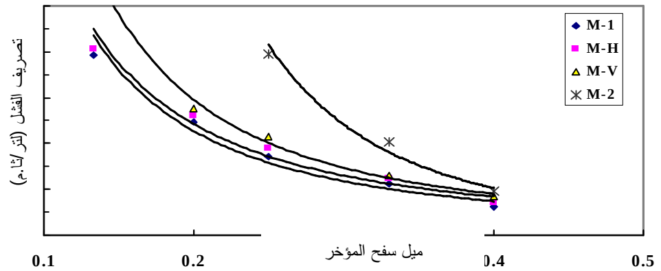
الشكل (5أ): العلاقة بين تصريف الفشل وميل سفح المؤخر لكتلة السلة الصخرية (1.510) كغم
