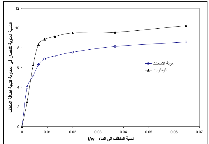
شكل رقم (2) تأثير المنظف على مقاومة الانضغاط لمونة السمنت والخرسانة
