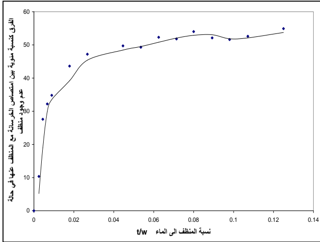
شكل رقم (3) تأثير نسبة المنظف على امتصاص الخرسانة
